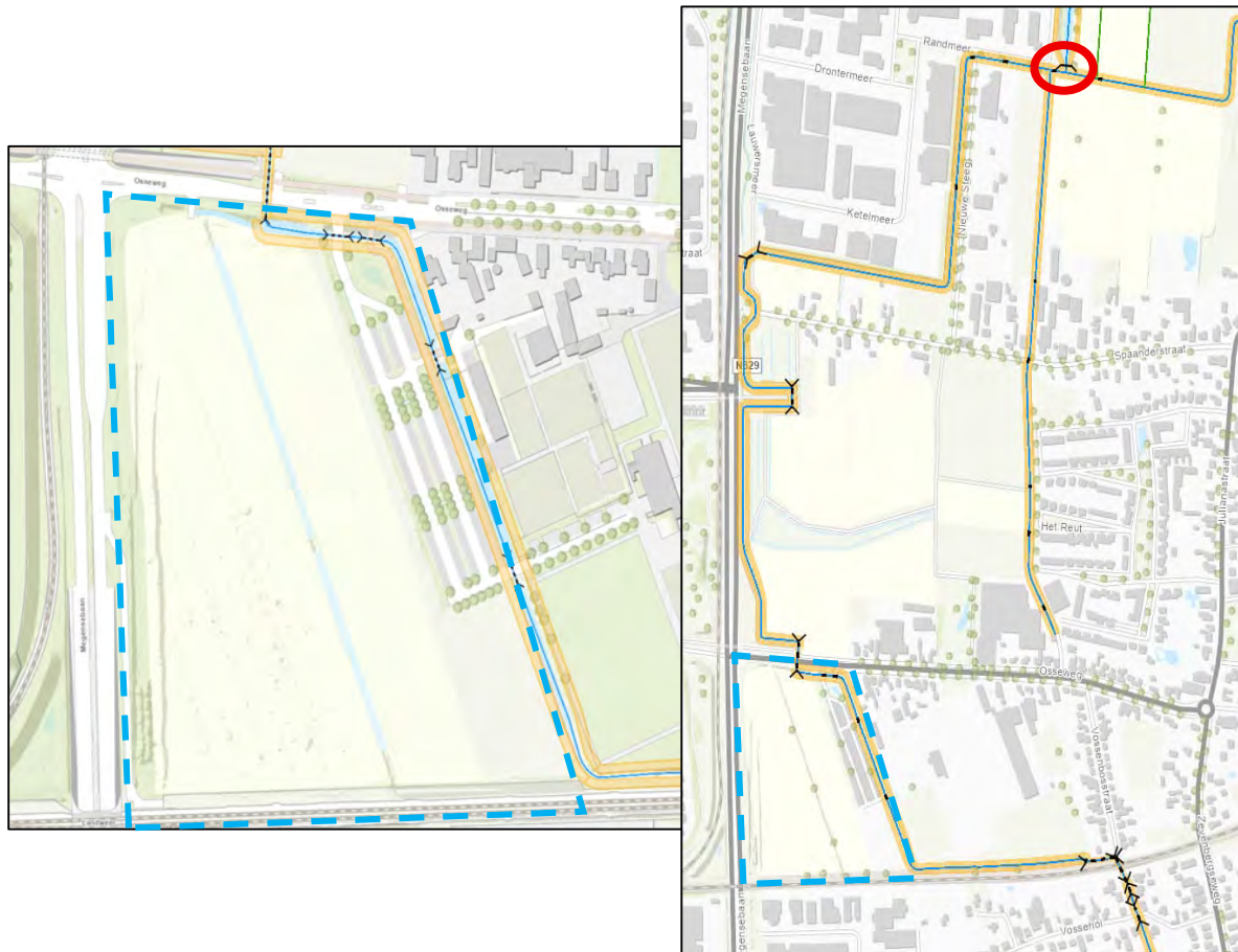
Figuur 4 projectgebied met oppervlaktewater dat via vrij verval wordt afgevoerd. Ten noorden van het gebied ligt een stuw (rood omcirkeld) waarachter zich wel een winter- en zomerpeil bevindt.
