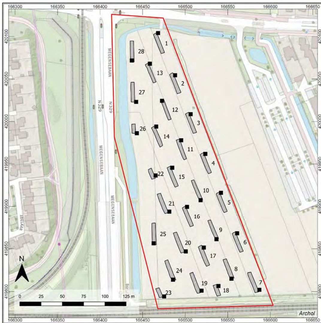
Figuur 2.2 Puttenkaart met de locaties van de gedocumenteerde profielen (zwart) binnen het onderzoeksgebied (rood).
