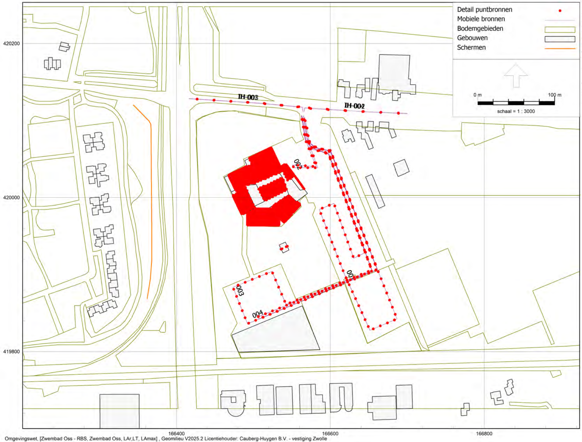
Figuur 3: Mobiele geluidbronnen
