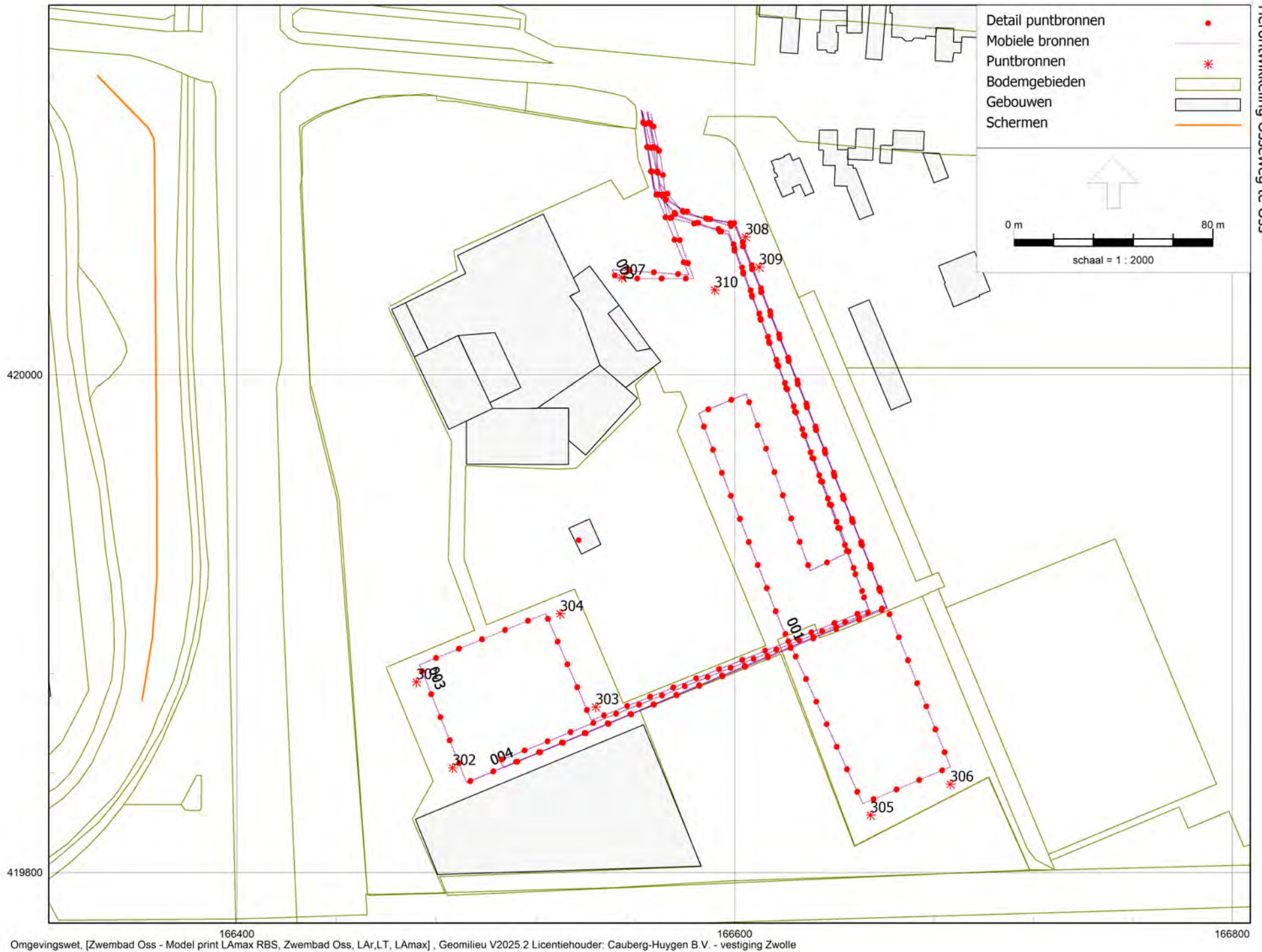
Figuur 4: Geluidbronnen maximaal geluidniveau
