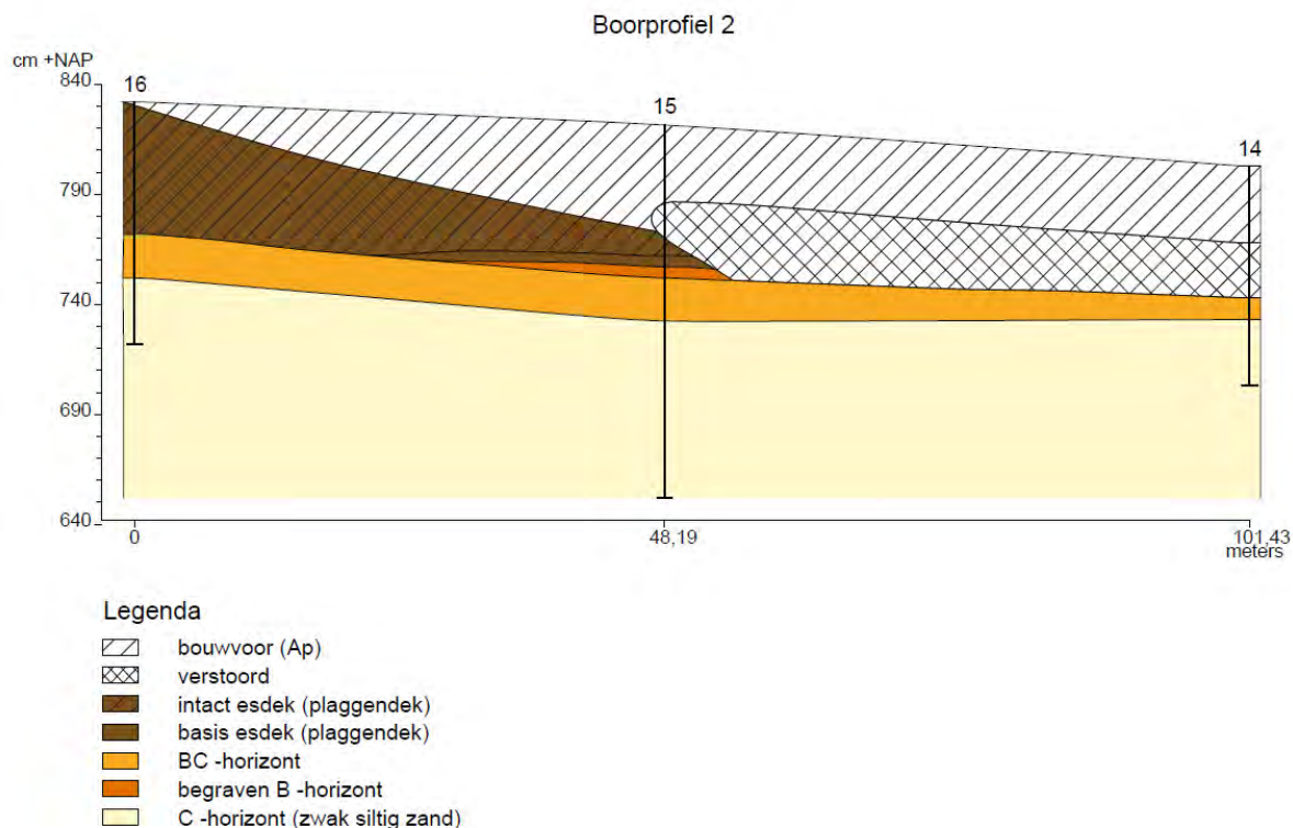
Figuur 3.5 Boorprofiel 2 met doorsnede van het onderzoeksgebied van west (links) naar oost (rechts) uit het bureau- en booronderzoek (bron: Duivenvoorden 2021, bijlage II).
